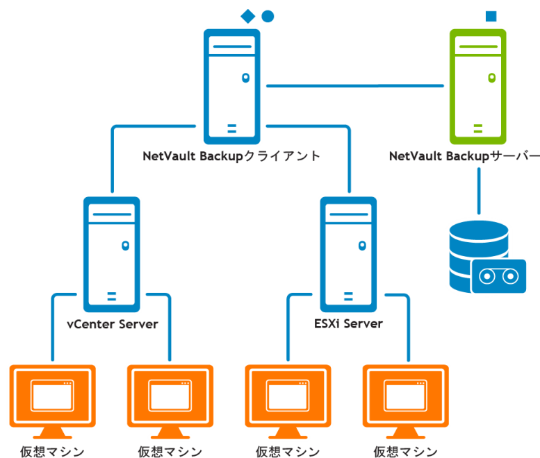
図 1. Plug-in for VMware システム構築例
